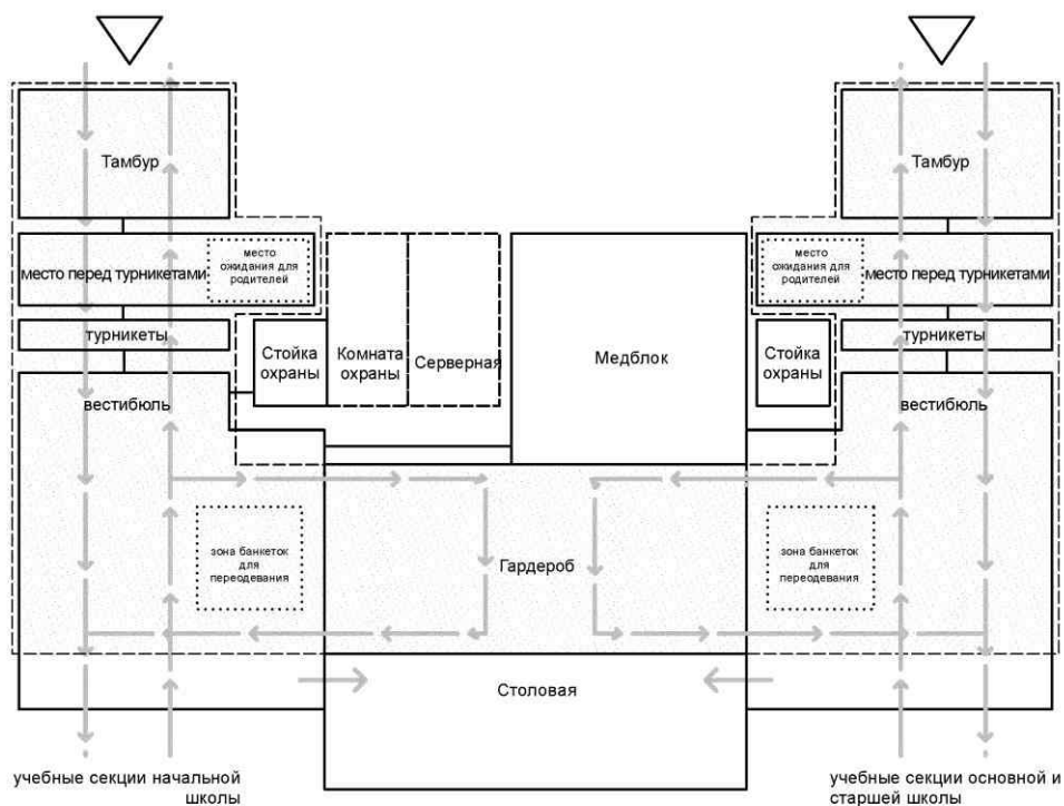
В. Децентрализованный вход
