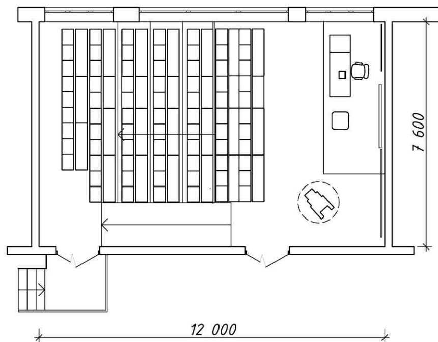
Рисунок 9 – Схема устройства потоковой аудитории с уклоном пола
