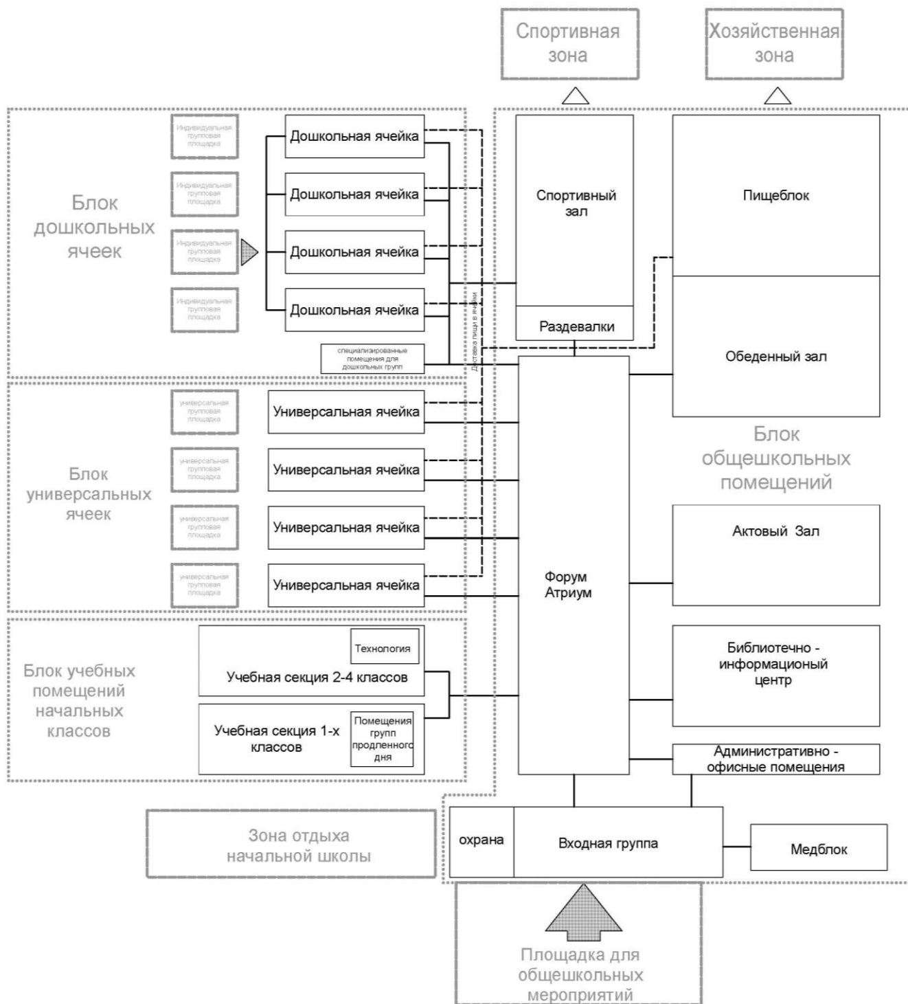
Рисунок 15 – Схема функционального зонирования комбинированного БНК
