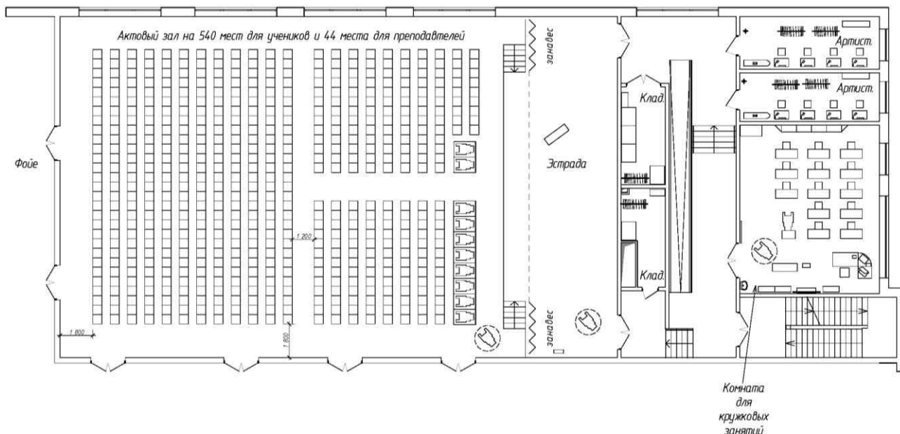
Рисунок 8 – Схема устройства актового зала, помещений при сцене, доступа МГН на сцену
