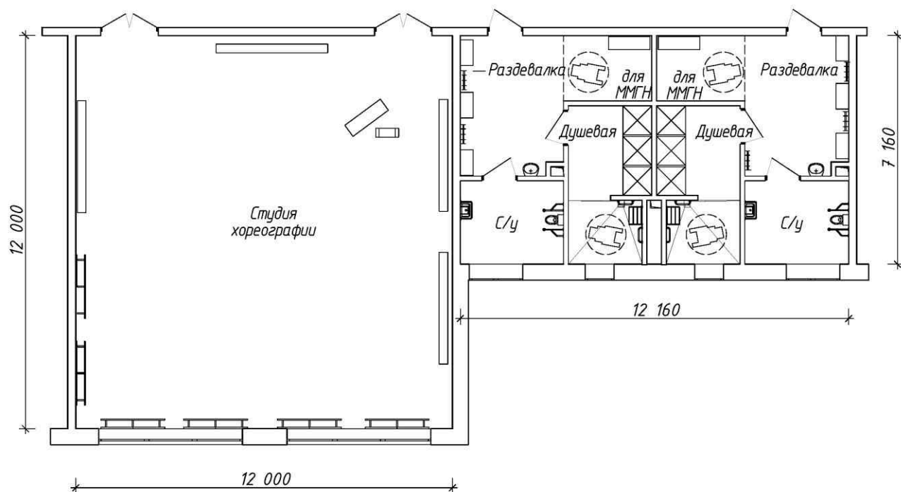
Рисунок 11 – Схемы спортивных залов
