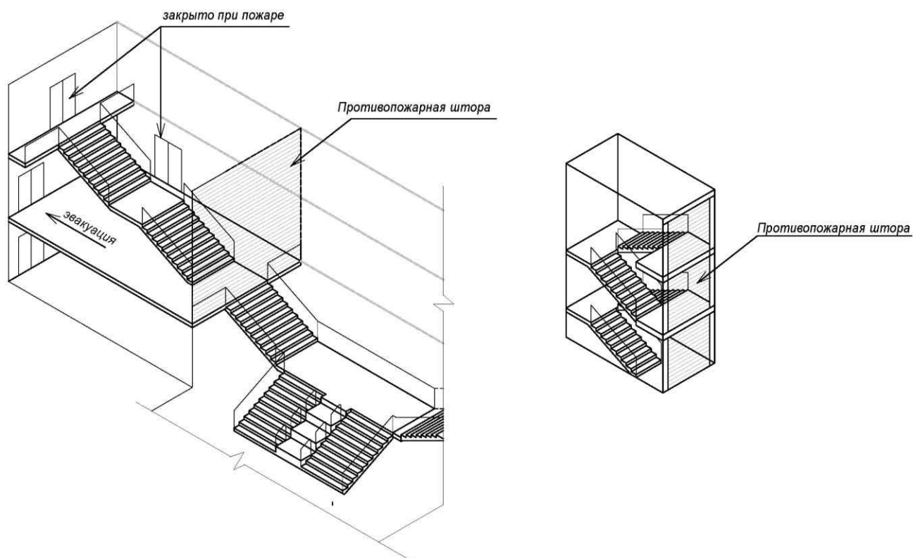
Рисунок 4 – Варианты устройства лестниц
