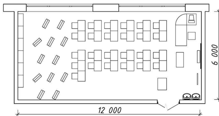
Рисунок 10 – Кабинет искусства. Схема размещения оборудования
