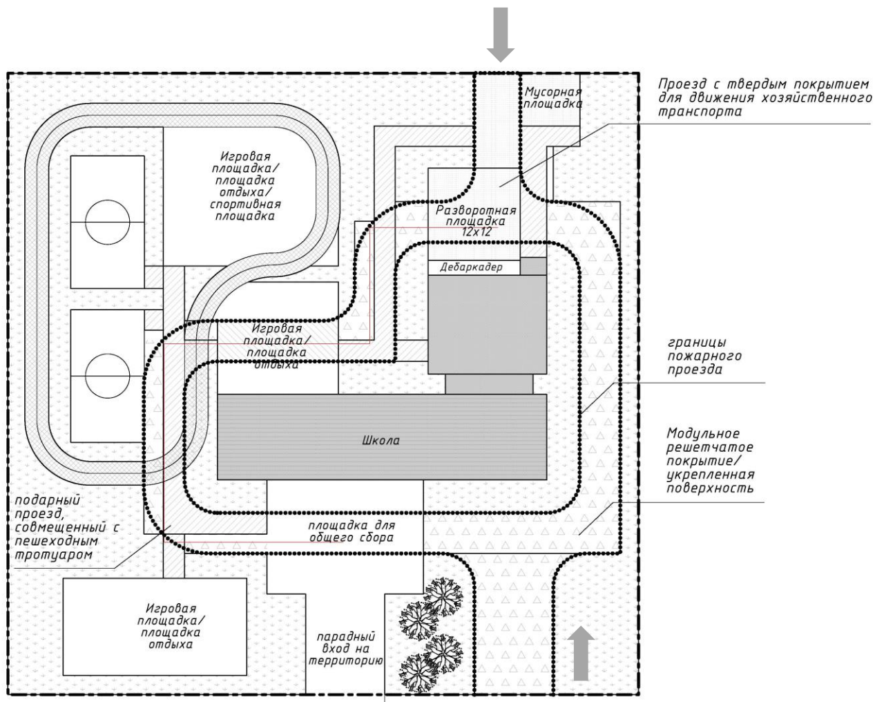
Рисунок 1 – Принципиальная схема организации пожарного проезда по территории ООО
